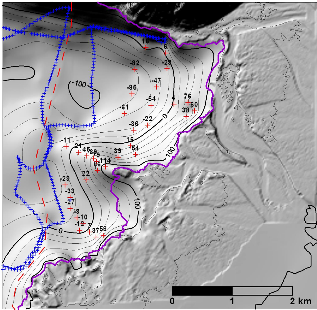
7. mynd. Botnhæðarlíkan felld við hæðarlíkan utan jökuls, sýnt sem skuggamynd og sem hæðarlínukort með 20 m á milli hæðarlína. Mæld botnhæð í nýju íssjárpunktunum er sýnd með rauðum krossum. Bláir krossar sýna staðsetningu eldri mælinga. Brotin rauð lína sýnir samskeyti við eldra botnlíkan (óbirt). Fjólublá lína sýnir jökuljaðar árið 2007.
