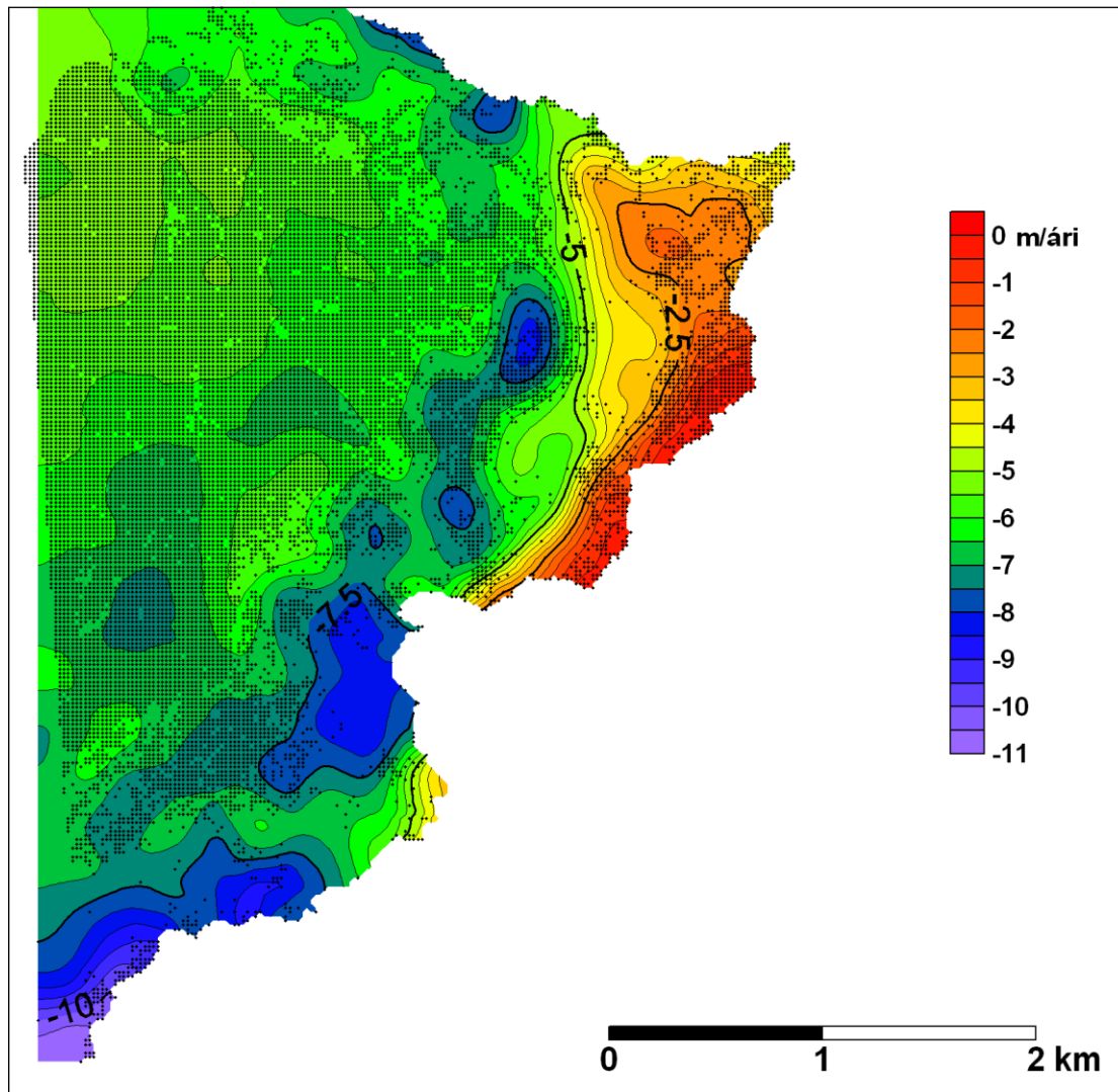
10. mynd. Meðalyfirborðslækkun á ári frá 2003 til 2007. Aðeins er sýnt það svæði þar sem enn var jökull árið 2007. Svörtu punktarnir sýna þau svæði þar sem hæðarmæling er til frá 2007, en brúað hefur verið í eyðurnar.
