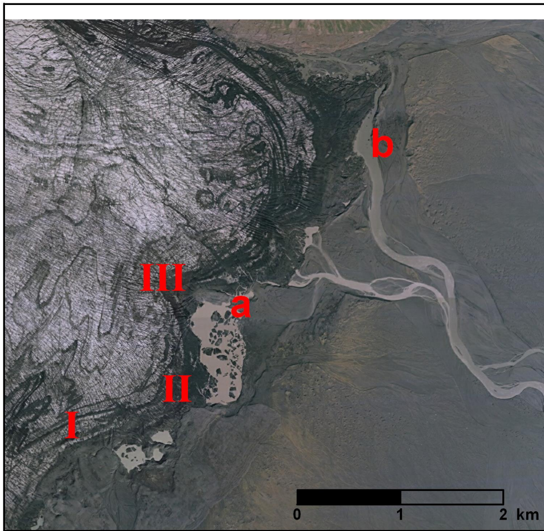
13. mynd. Þrjú jökulhöft milli lóna og útfalla Skeiðarár ( I-III ) sem halda aftur af rennsli í vesturátt. Einnig er merkt inn á sandhryggur ( a ) og núverandi meginútfall Skeiðarár.
