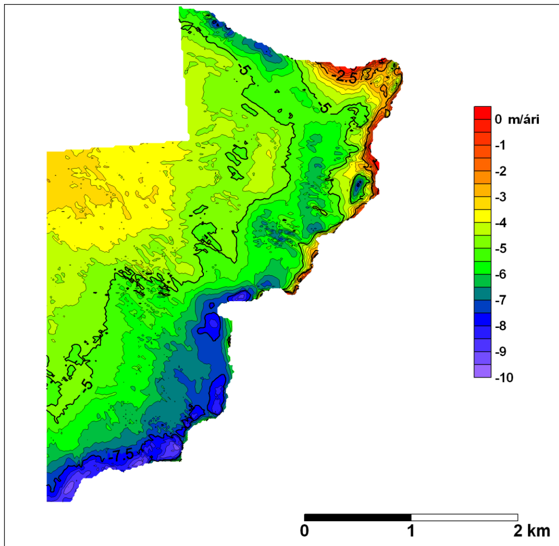
9. mynd. Meðalyfirborðslækkun á ári frá 1997 til 2003. Aðeins er sýnt það svæði þar sem enn var jökull árið 2003.
