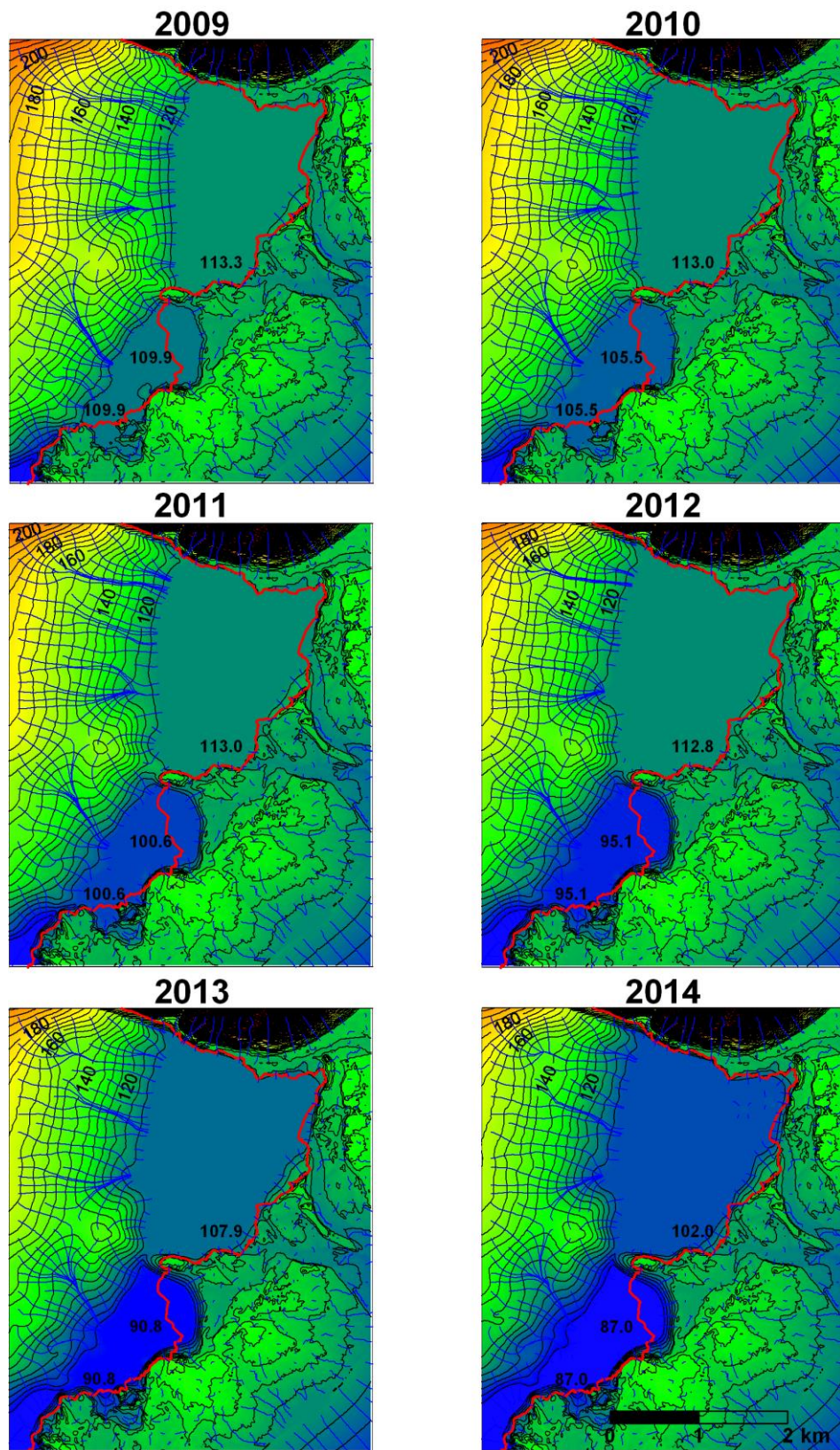
12. mynd. Vatnsmættishæð (svartar jafnhæðalínur) og rennslisleiðir (bláar) fyrir fargstuðul k = 0.9 , áætlað fyrir árin 2009-2014. Hæð jaðarlóna og mættispolls austast á jöklinum er merkt sérstaklega. Jaðar frá 2007 (rauður) er sýndur til viðmiðunar.
