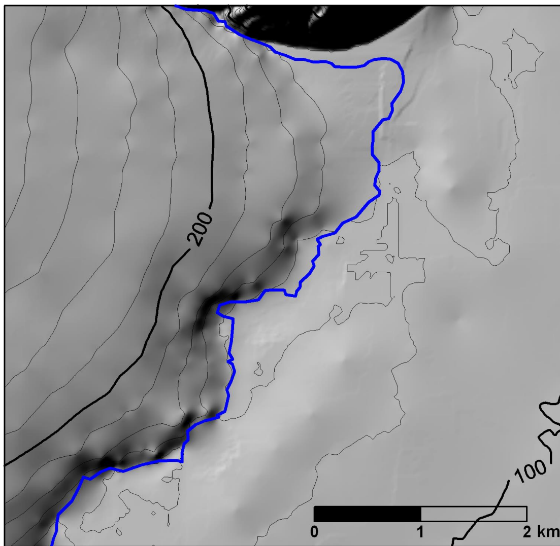
5. mynd. Hæðarlíkan af rannsóknasvæði byggt á hæðarlínum hnituðum af korti Loftmynda ehf. af Skaftfelli og nágrenni frá 2003, sýnt sem skuggamynd og sem hæðarlínukort með 20 m á milli hæðarlína. Jökuljaðar frá 2003 er sýndur sem blá lína.
